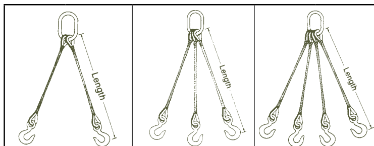
2-Leg Bridle
